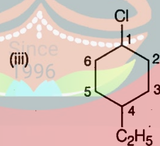
1-क्लोरो-4-एथिलसाइक्लोहेक्सेन
