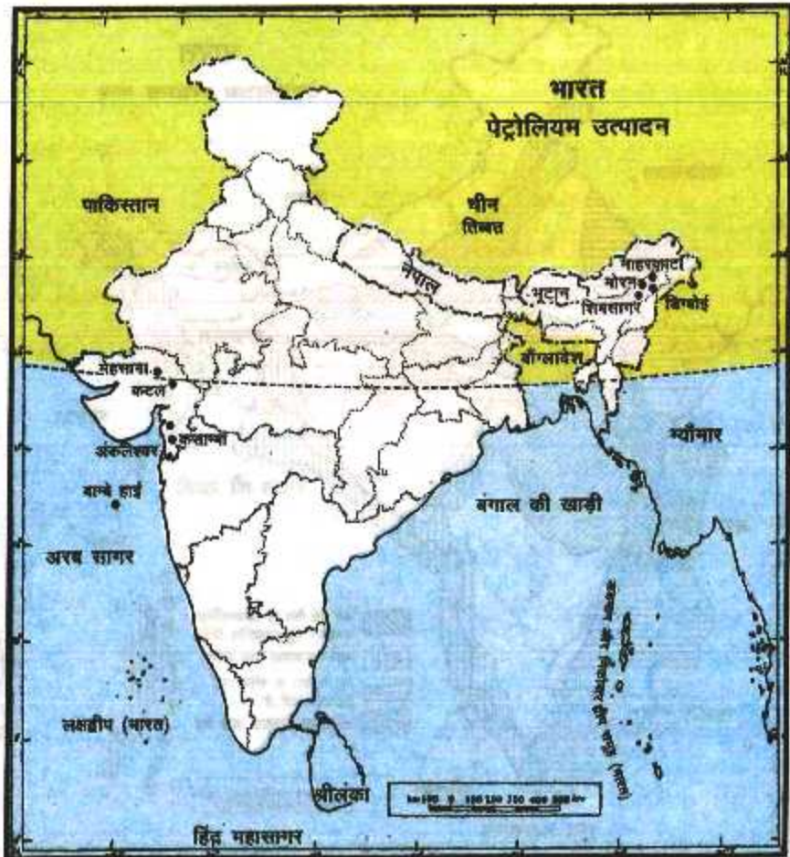
चित्र-1 (ड).5 : भारत में पेट्रोलियम उत्पादन क्षेत्र
